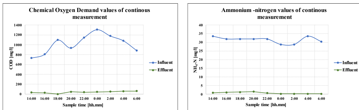
Figure 5. COD and \text{NH}_4\text{-N} values over the continuous measurements 5. ábra. A \text{COD} és \text{NH}_4\text{-N} értékek változása az automata mintavevővel történt mérés során
