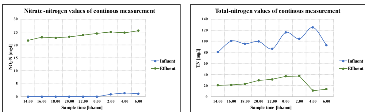
Figure 6. \text{NO}_3 and TN values over the continuous measurement 6. ábra. A \text{NO}_3 és \text{TN} értékek változása az automata mintavevővel történt mérés során
