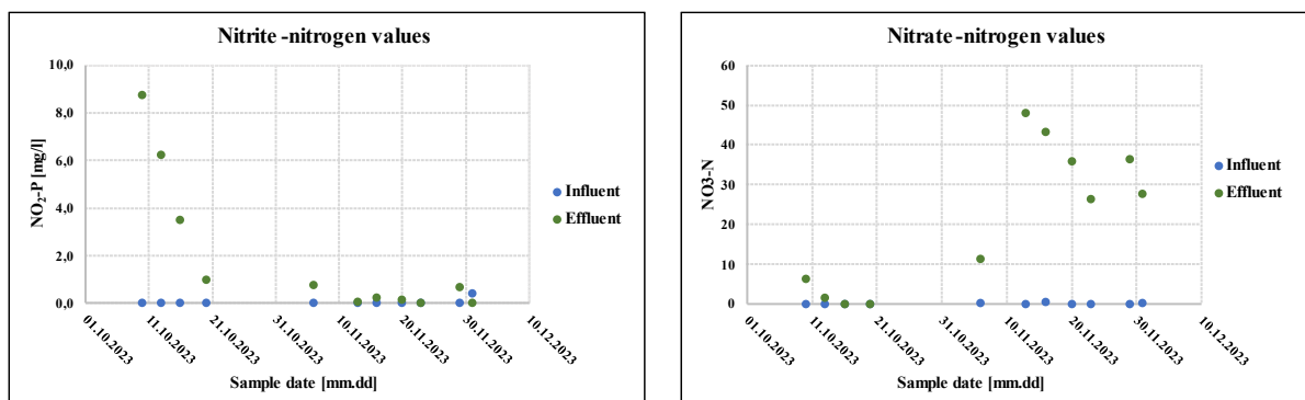
Figure 4. \text{NO}_2\text{-N} and \text{NO}_3\text{-N} values over the experiment 4. ábra. A \text{NO}_2\text{-N} és \text{NO}_3\text{-N} értékek változása a kísérlet során
