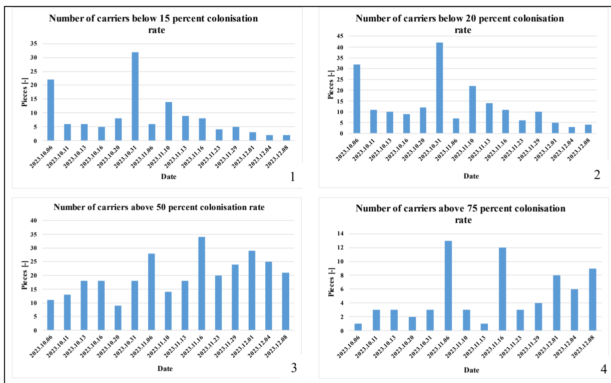
Figure 9. Number of carriers according to the colonisation rate 9. ábra. Mikrohordozók száma betelepültség függvényében
