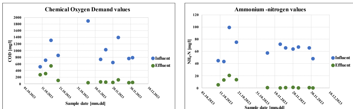
Figure 3. COD and \text{NH}_4\text{-N} concentration of inflow and effluent during the biofilm development process 3. ábra. A KOI és \text{NH}_4\text{-N} koncentráció változása a be- és elfolyóban a betelepülés során
